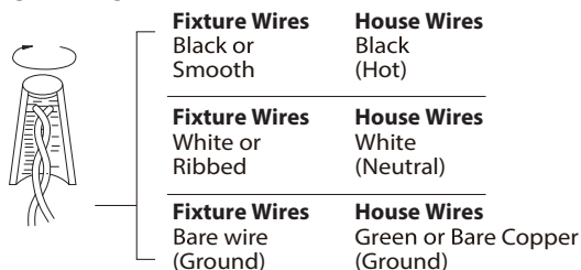
Fig. 2 Wiring
