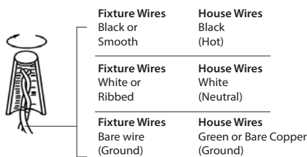
Fig. 2 Wiring
